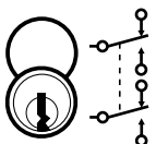
Key pos. 1 Swt. pos. 1
