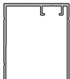
011007 Binario superiore 1via Upper rail 1 way
