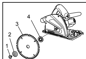
1. Boulon hexagonal 2. Bague externe 3. Lame 4. Bague interne
