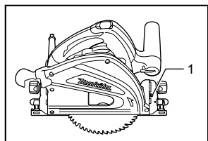
1. Vis de réglage 45°
