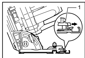
1. Levier coulissant
