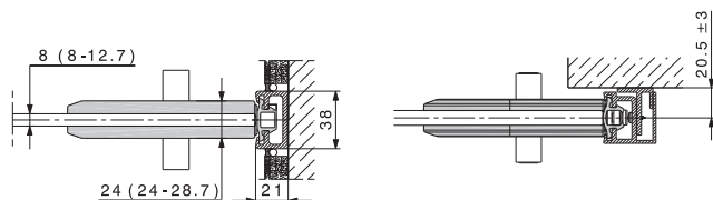
Montaje mural
