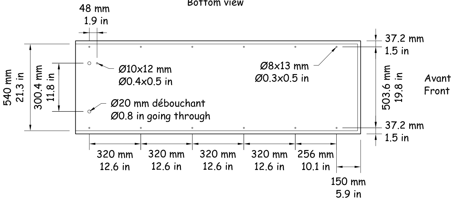
Vue de dessous Bottom view
