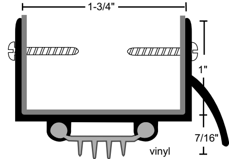
319V 319VDKB
