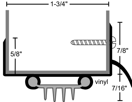
319EV 319EVDKB
