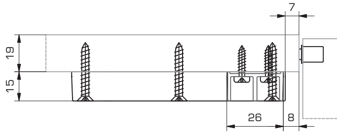
Aufgesetzte Führung Surface-mounted guide Guidage en applique
