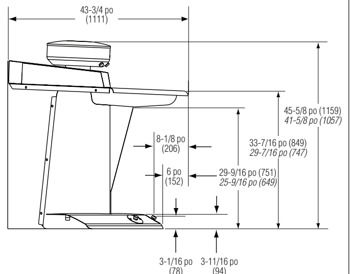
Unité à montage mural à commande à main
