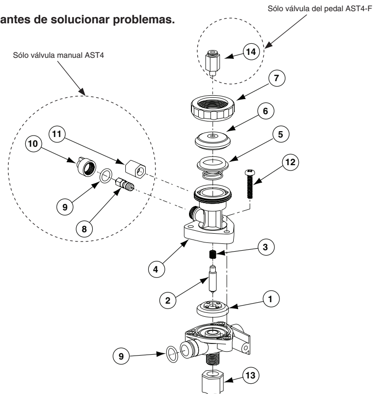
Válvula manual AST4, válvula del pedal AST4-F
