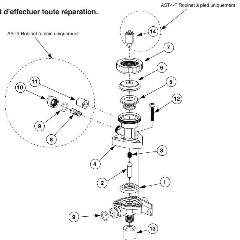
AST4-Robinet à main, AST4-F Robinet à pied
