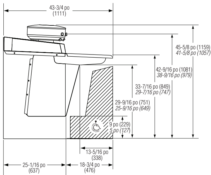
Unité à montage mural à commande à main
