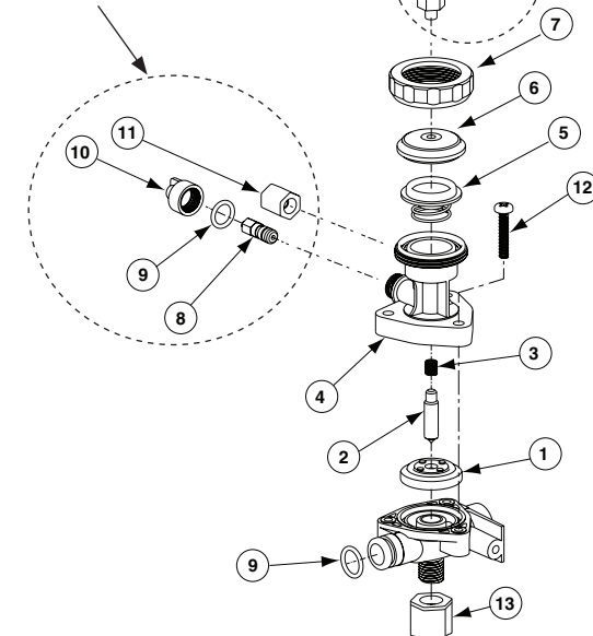
Válvula manual AST4, válvula del pedal AST4-F
