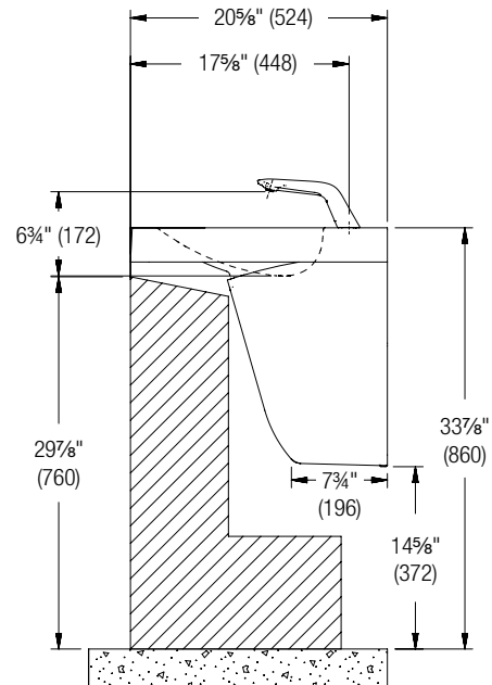
CSA Height – WBD1
