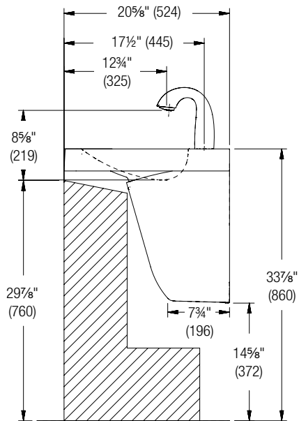
CSA Height – Verge Faucet
